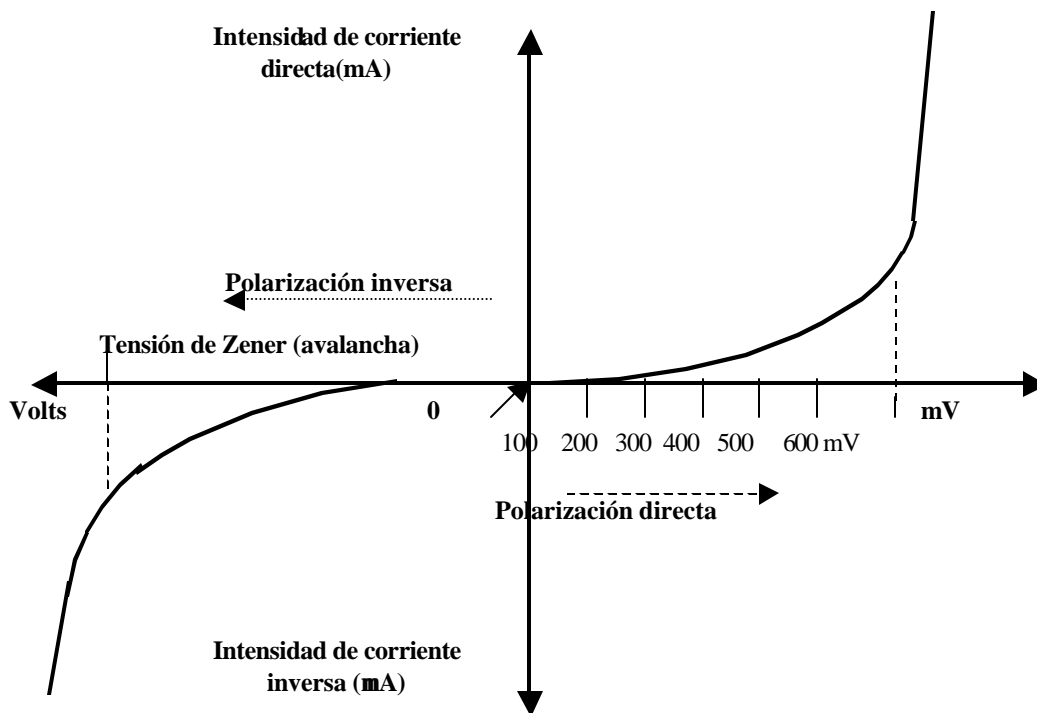
Fig. 12 - Curva característica Tensión de Polarización vs. Corriente de una juntura P-N
