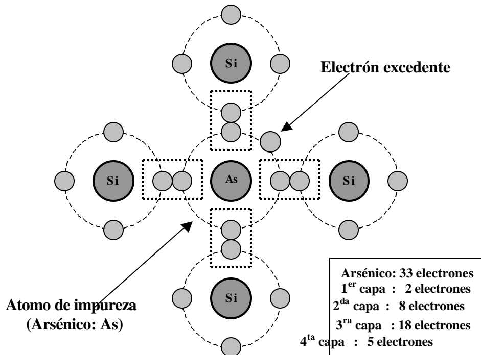
Fig. 7 – Material tipo N
