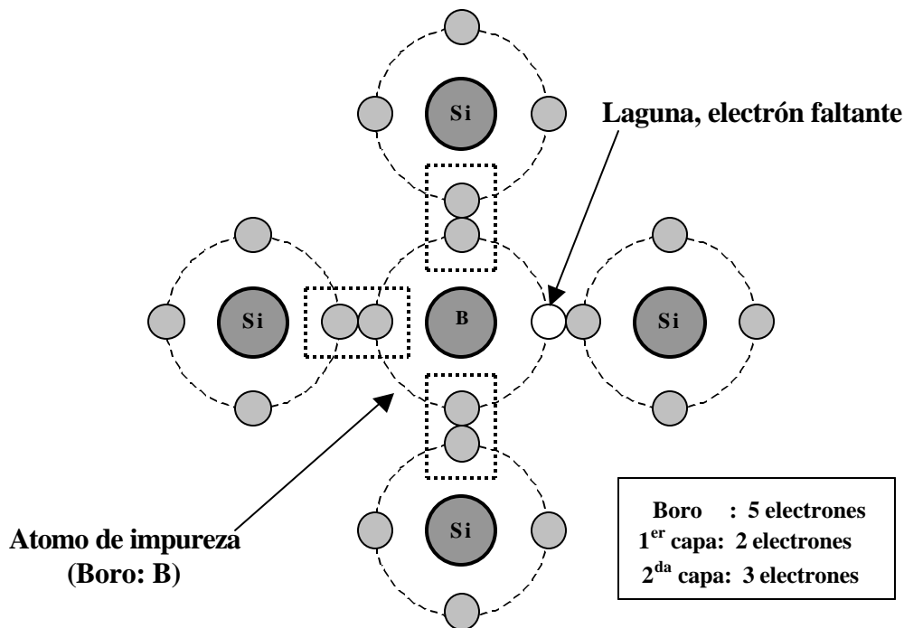
Fig. 8 – Material tipo P
